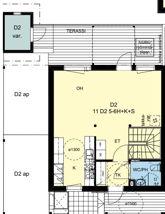
1. kerros 1:100
